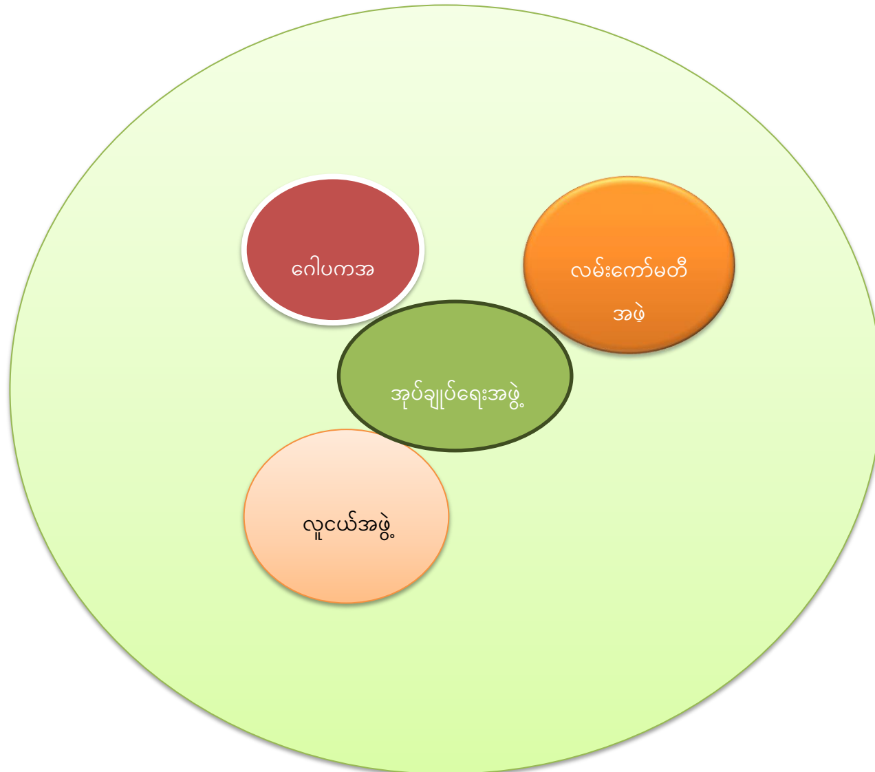
Venn Diagram
